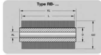
Барабанная стандартного исполнения
