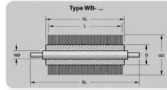
Роликовая стандартного исполнения
